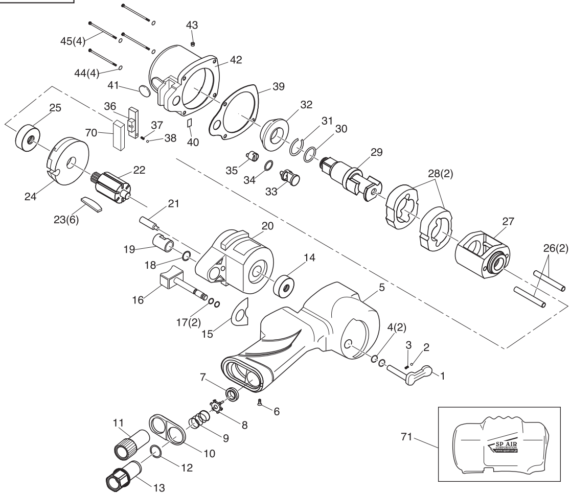
分解図
