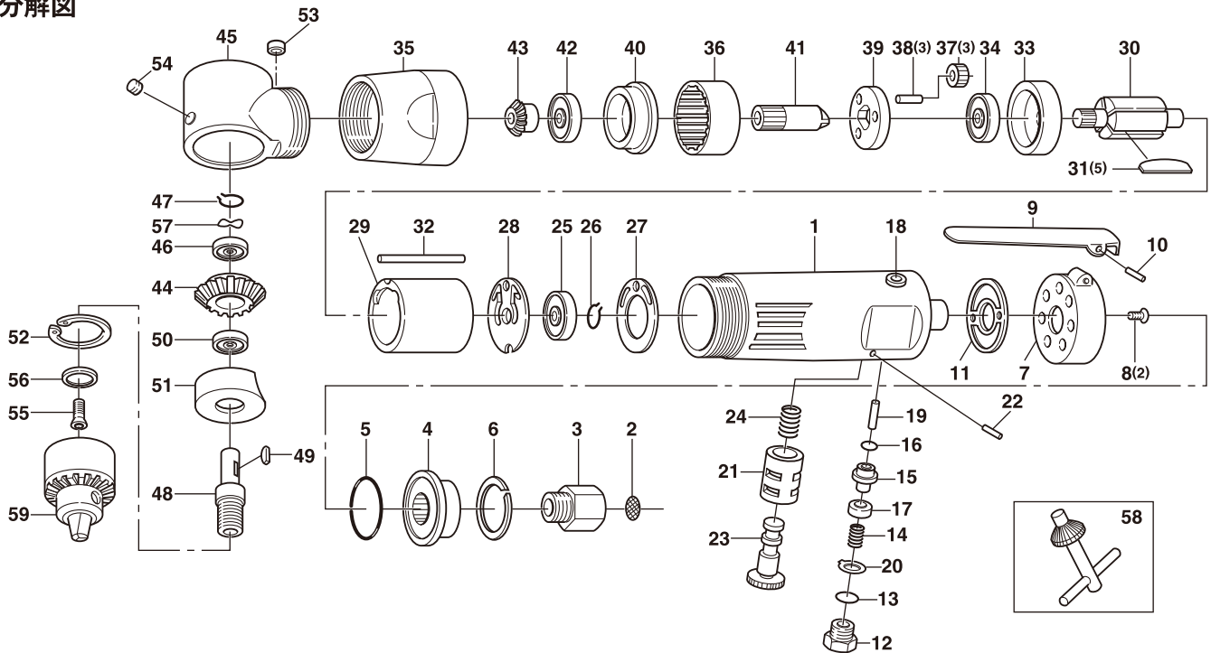
分解図
