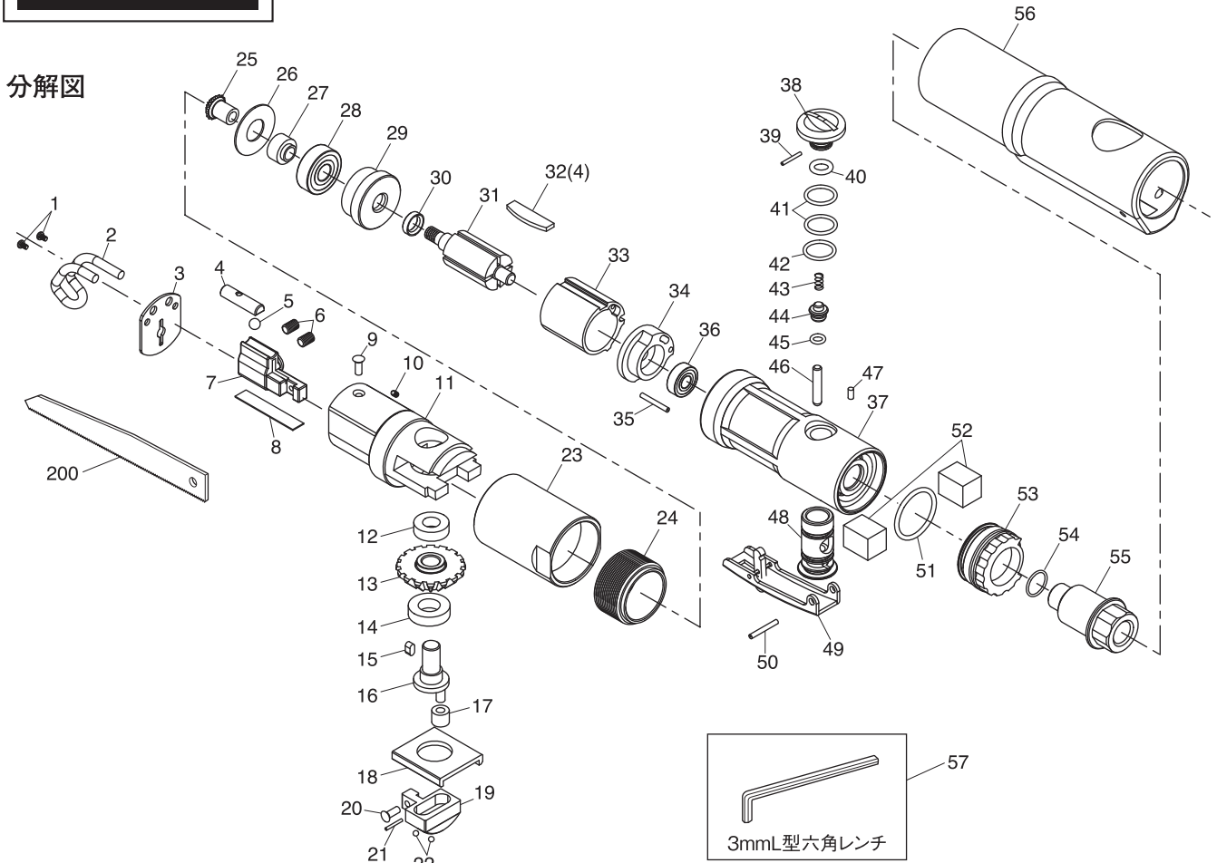
分解図
